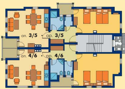
етажи 2/3 • floors 2/3
