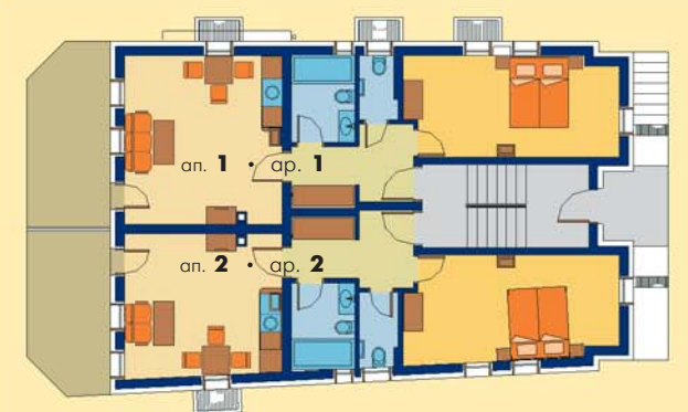
етаж 1 • floor 1
